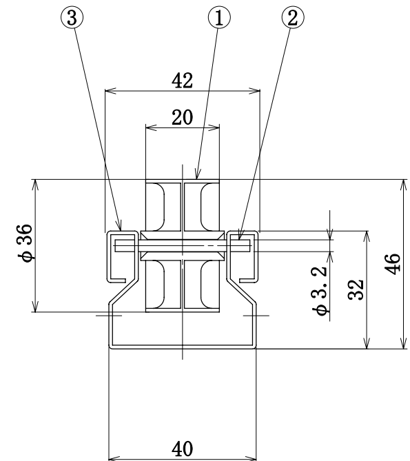
断面詳細
