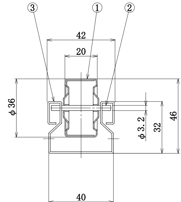
断面詳細
