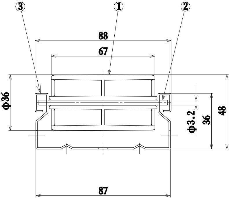
断面詳細
