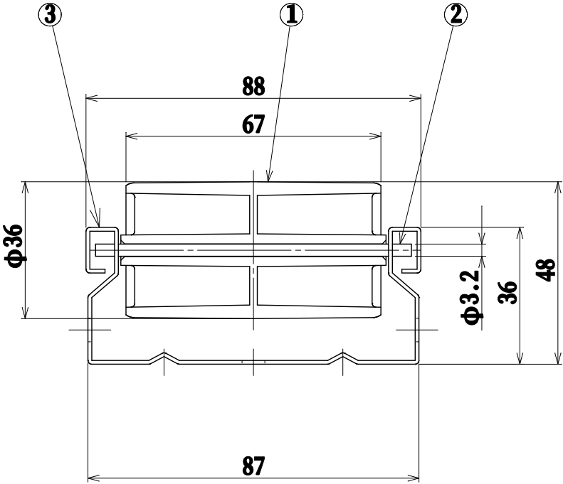
断面詳細
