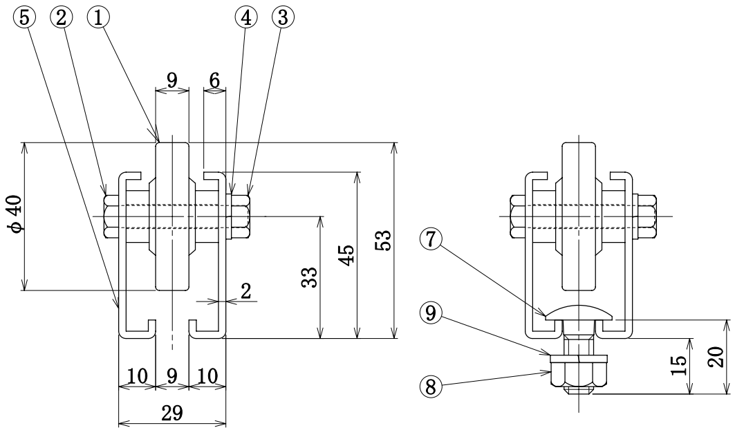
断面詳細
