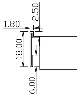
棚板開口部断面拡大図
