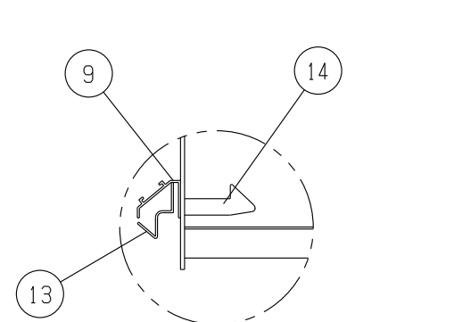
飛び出し防止機構A部詳細 ( S = 1 / 5 ) ※引き手キャップを外した状態 A部詳細 ( 1 / 7 )
