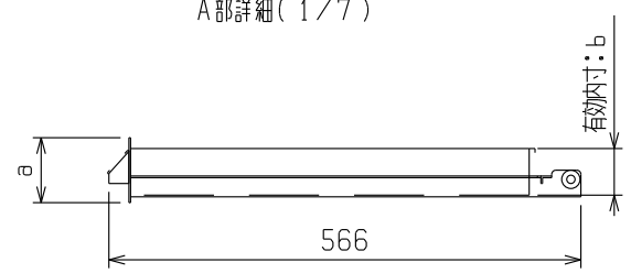
飛び出し防止機構A部詳細 ( S = 1 / 5 ) ※引き手キャップを外した状態 A部詳細 ( 1 / 7 )
