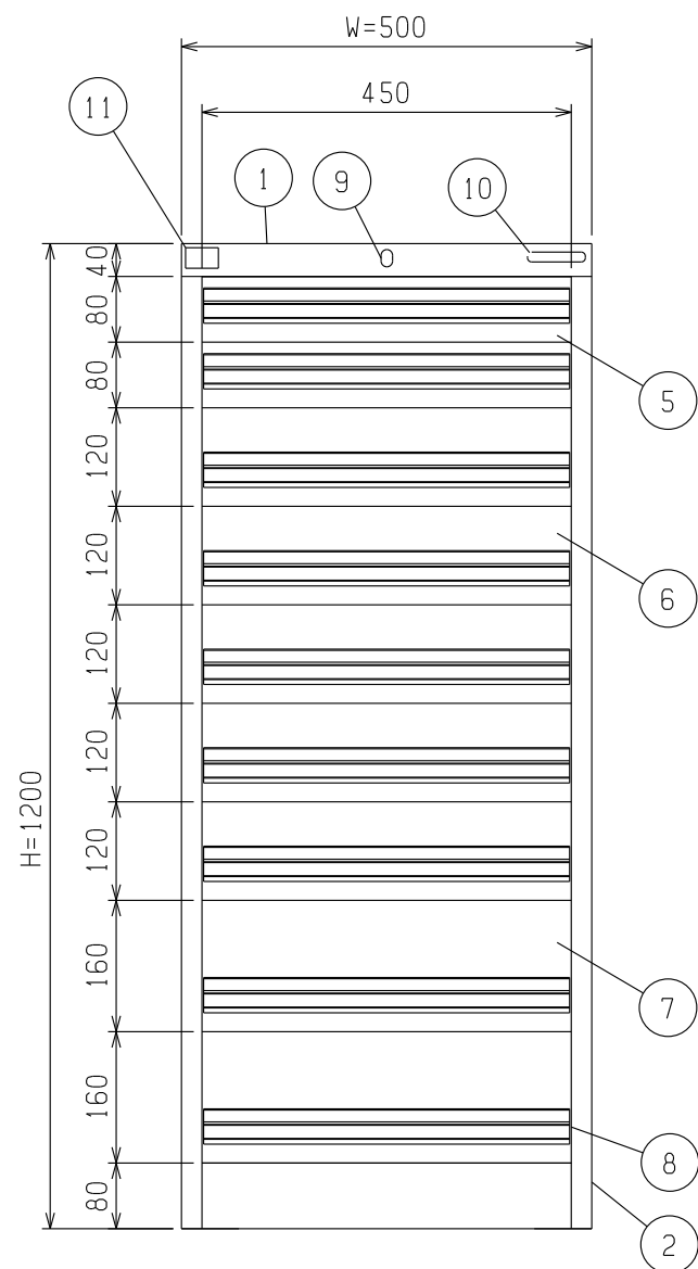
A部詳細( 1 / 7 )
