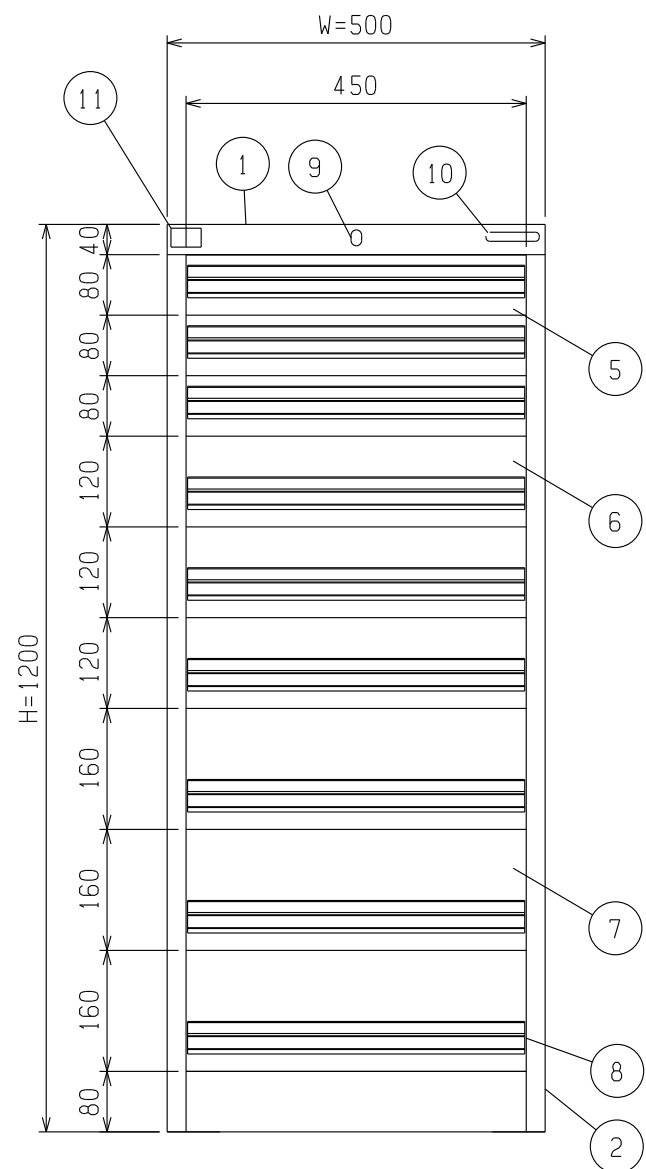
A部詳細( 1/7 )
