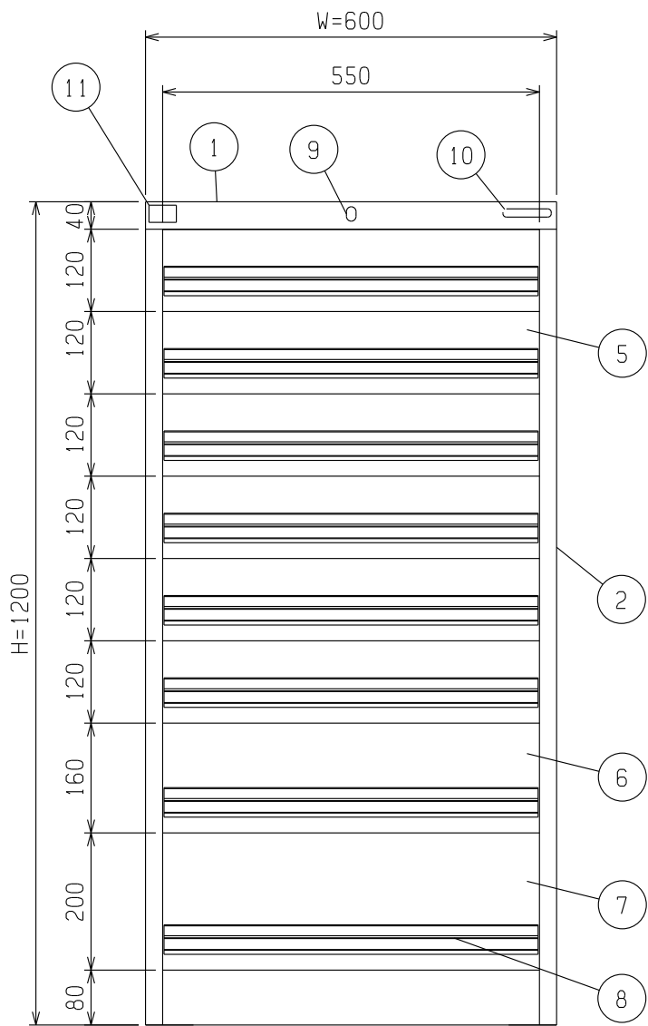
A部詳細 ( 1 / 7 )
