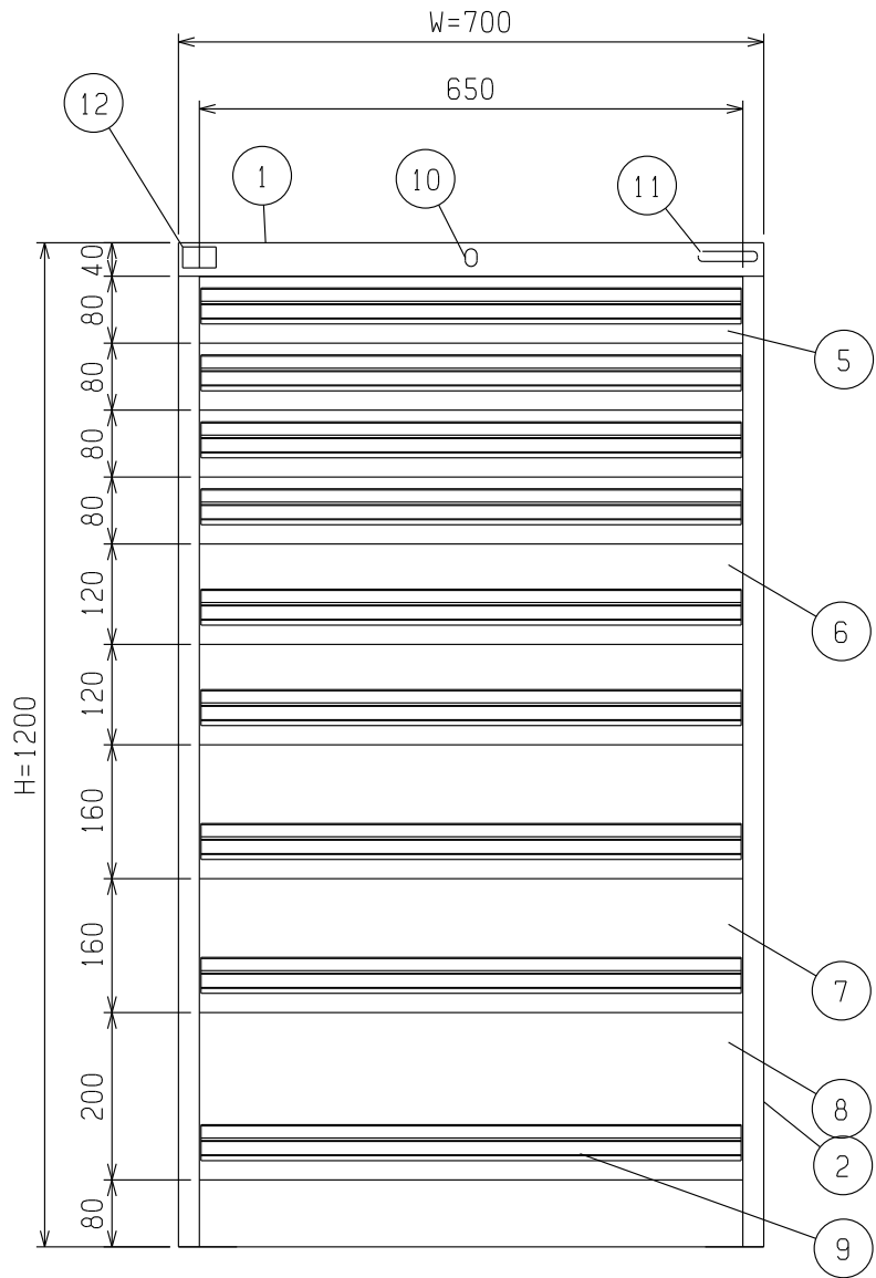
A部詳細( 1/7 )
