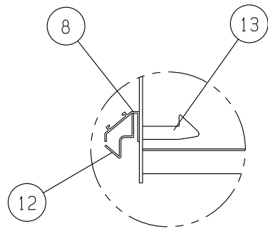
飛び出し防止機構A部詳細( S=1/5 )
