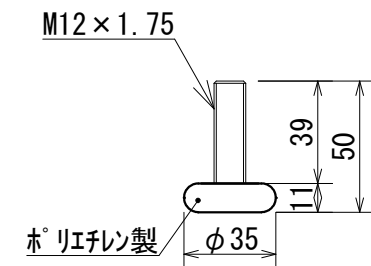
高さ調整レベル詳細 (1/2)
