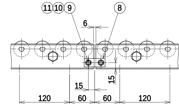
連結詳細
