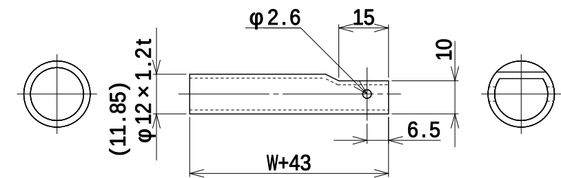
軸詳細
