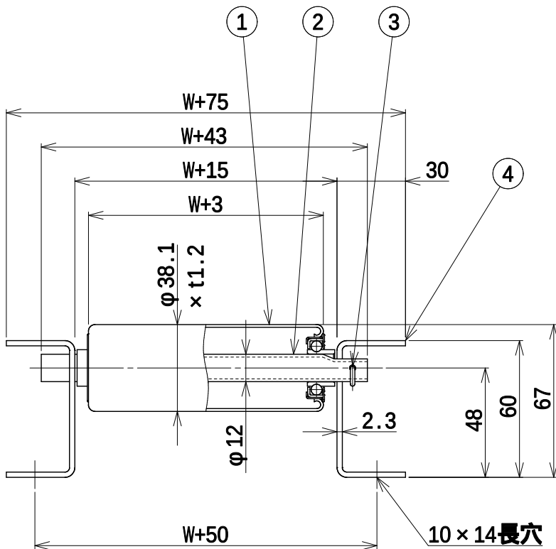
断面詳細
