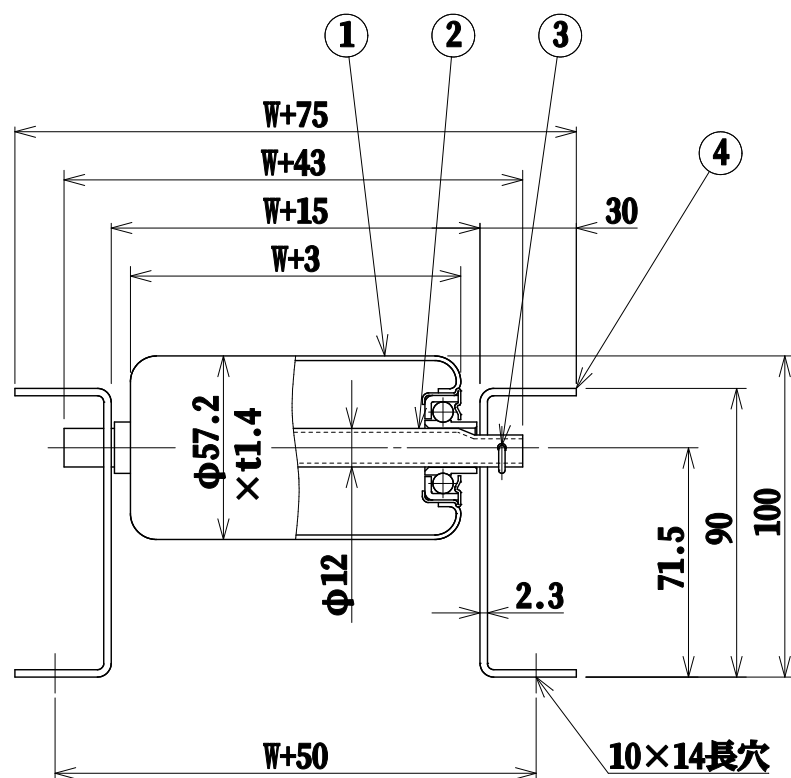
断面詳細
