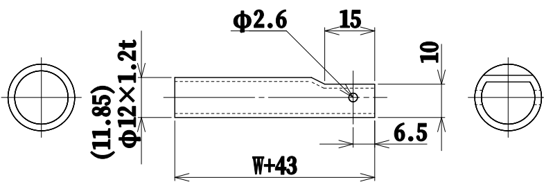
軸詳細
