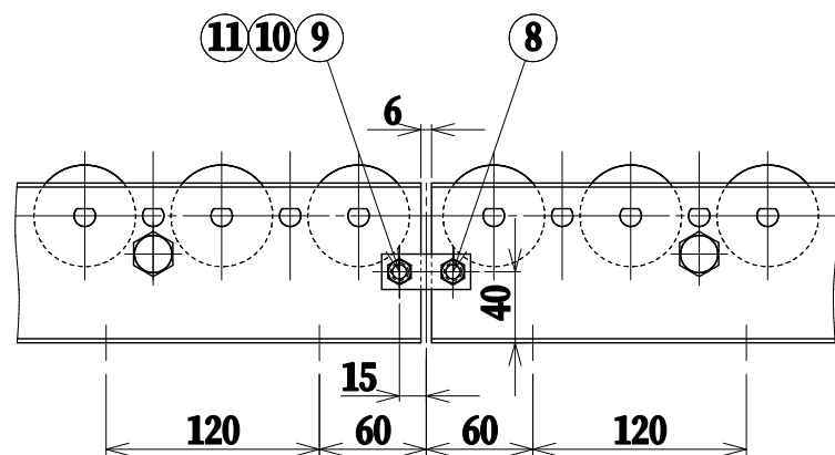
連結詳細
