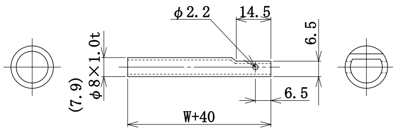
軸詳細
