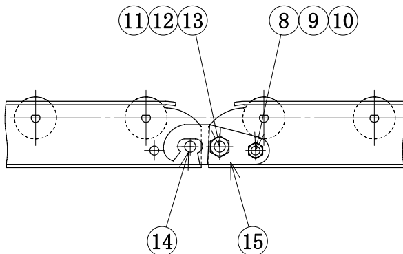
連結詳細
