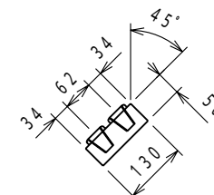
A - A 断面
