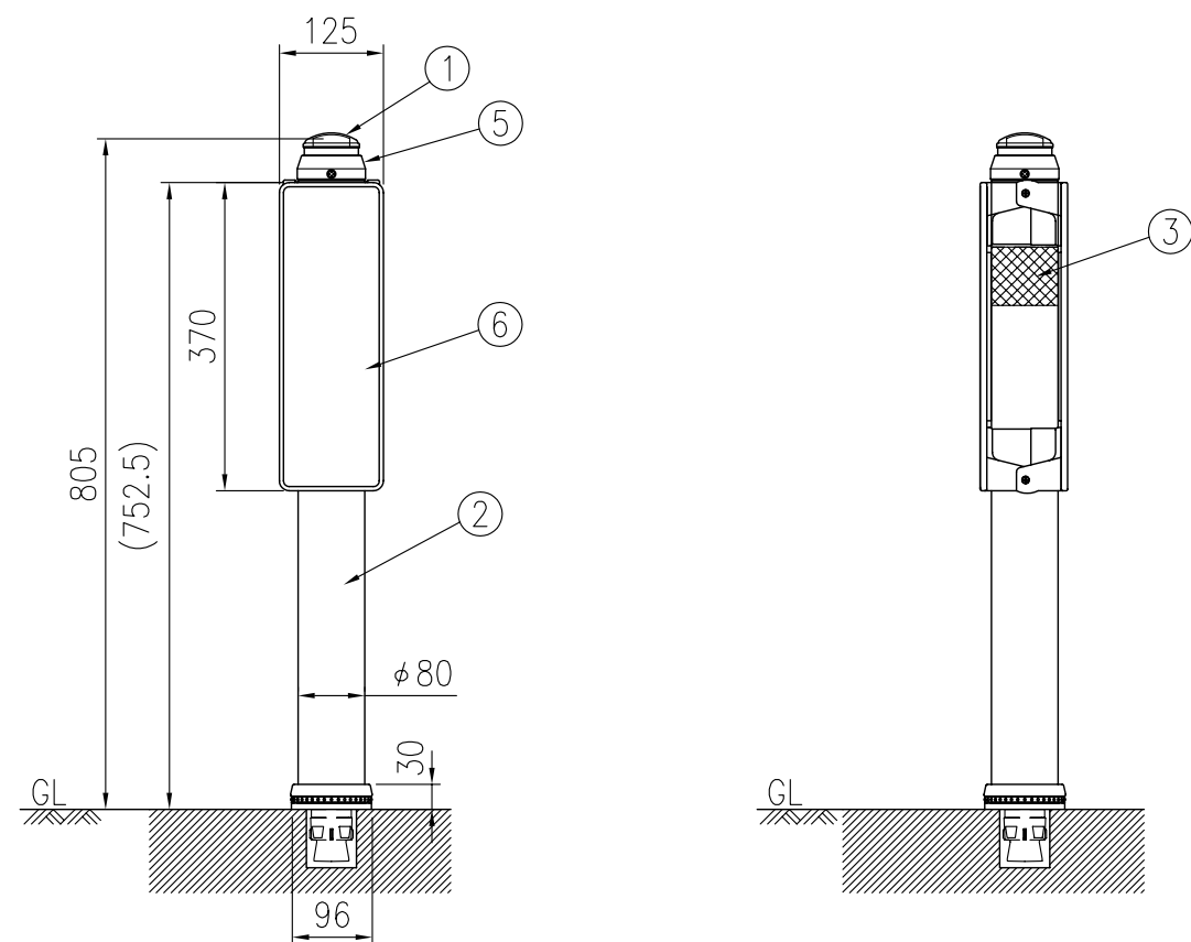
姿図 S=1/10
