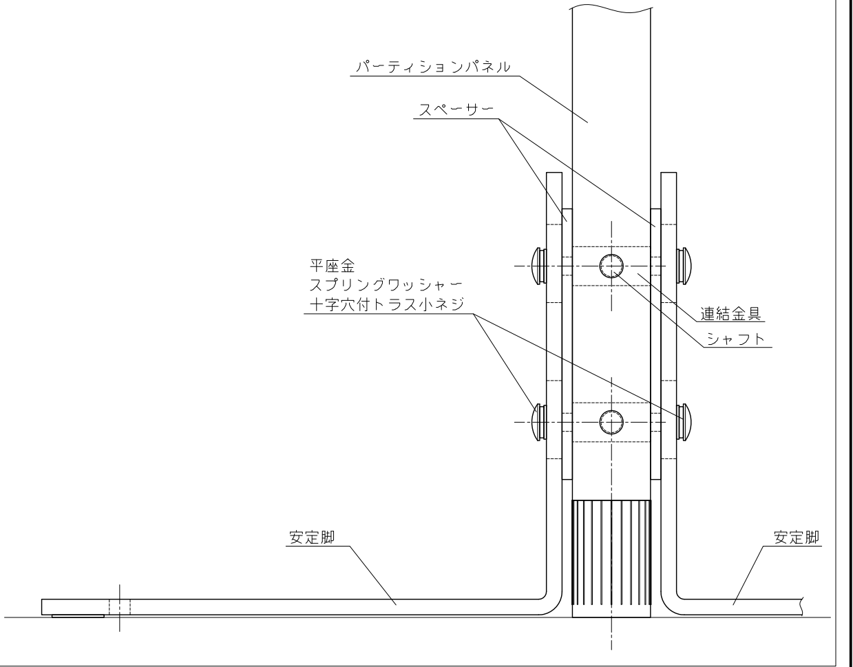
パネル組付図
