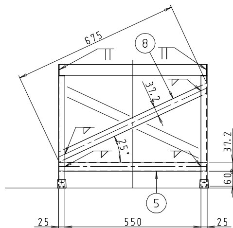
天板裏側溶接位置図
