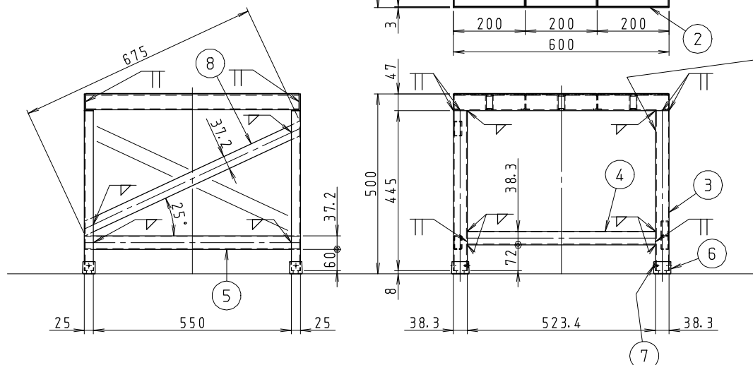
天板裏側溶接位置図
