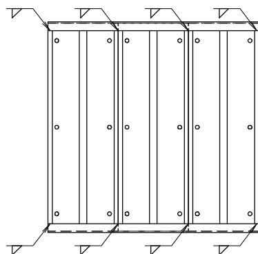
天板裏側溶接位置図
