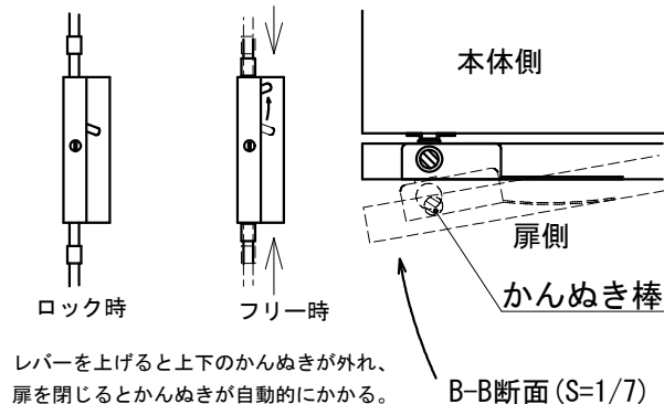
A部詳細 (S=1/7)
