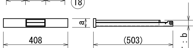
A部詳細 (S=1/7)
