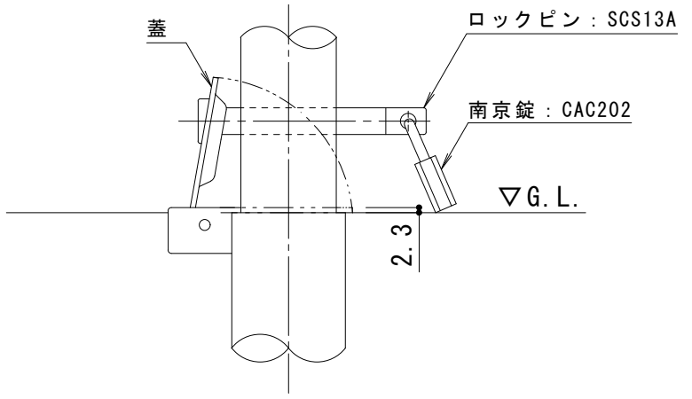
南京錠部詳細図 S = 1 : 3
