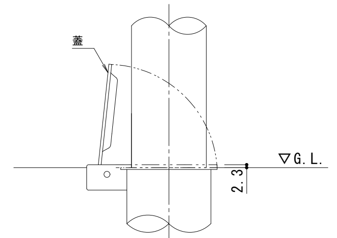
埋設管蓋部詳細図 S = 1 : 3
