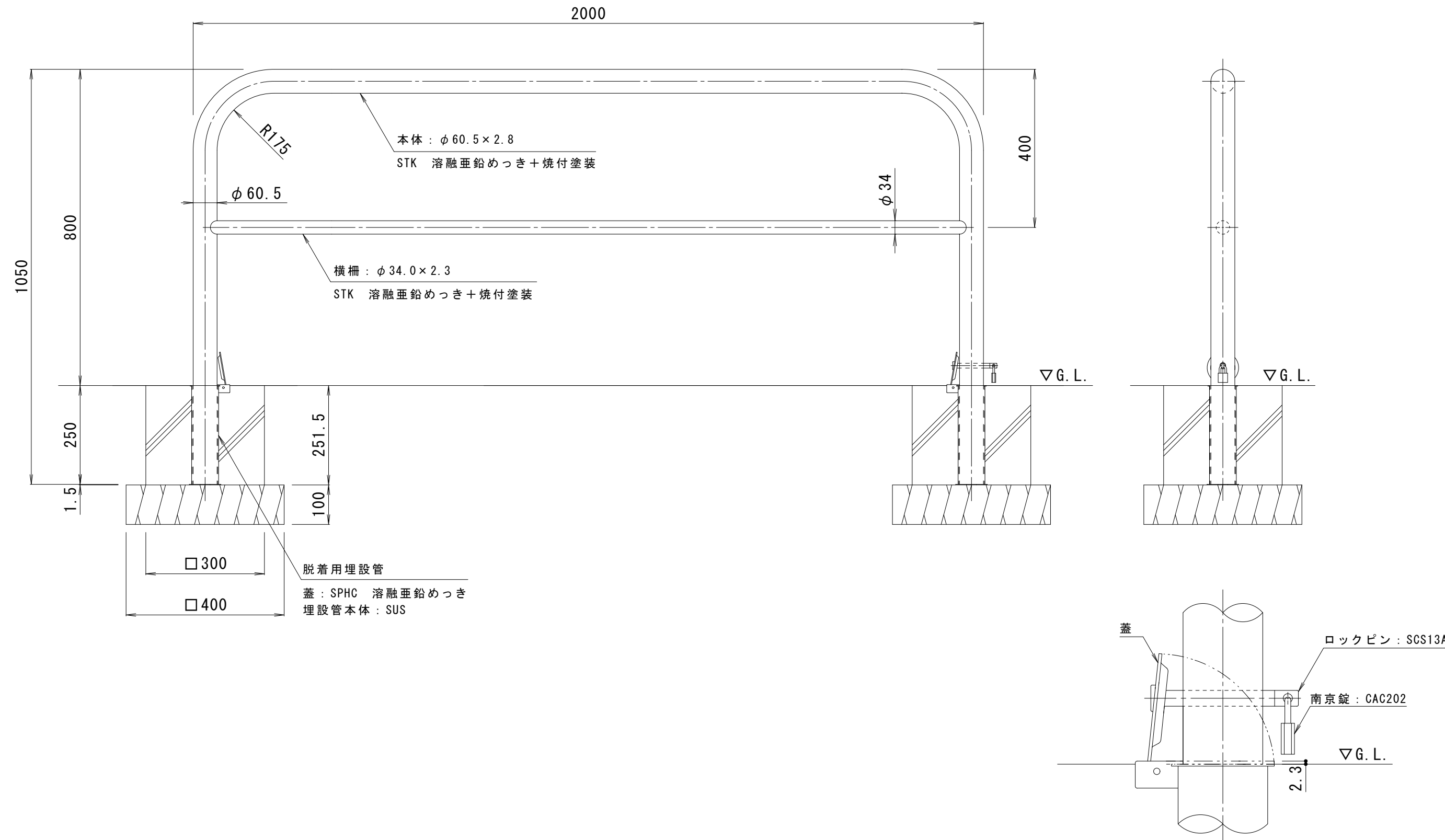
南京錠部詳細図 S = 1 : 3
