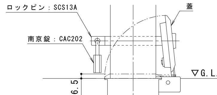
南京錠部詳細図 S = 1 : 3
