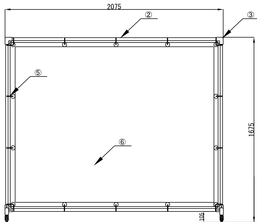
正面図
