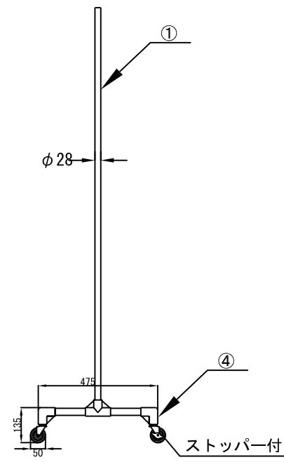
側面図
