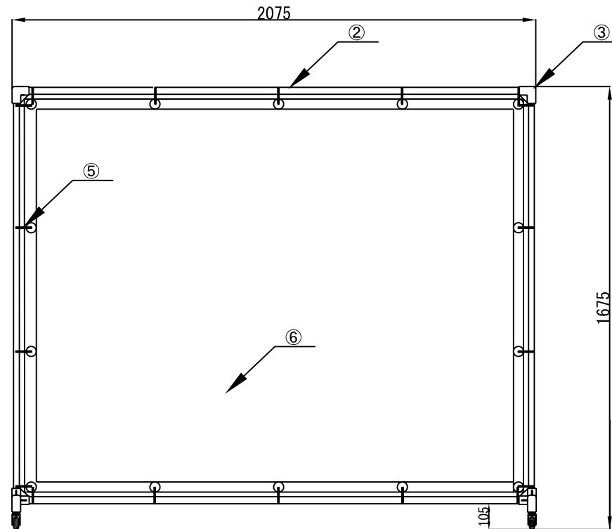
正面図
