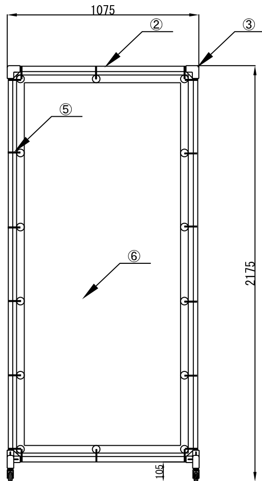
正 面 図
