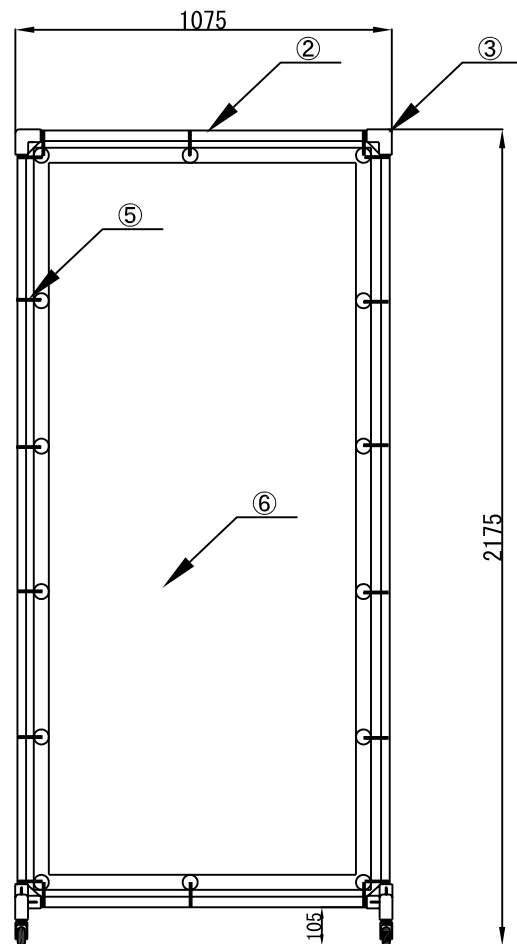
正面図
